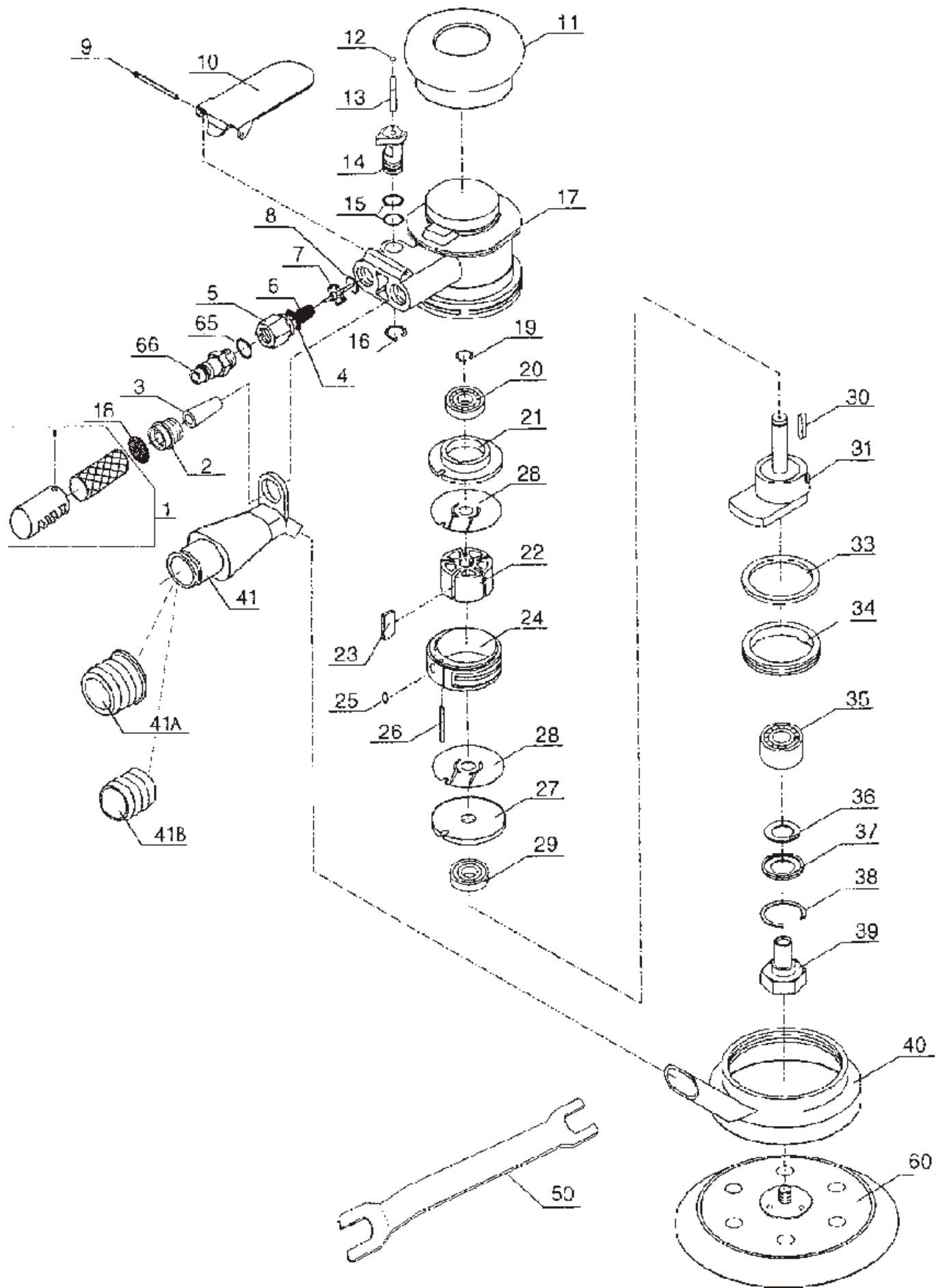
LEVIGATRICE PNEUMATICA CR 015 C
